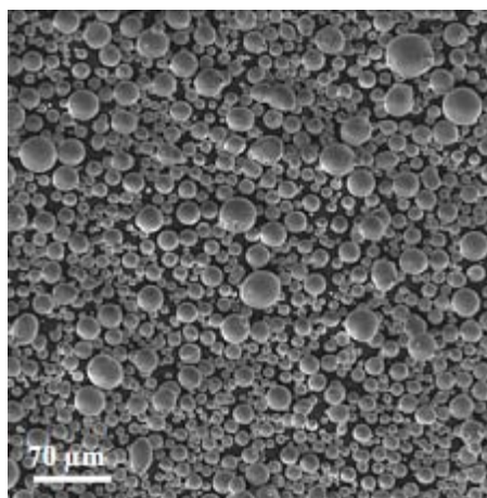
SEM of Zircox™ 3Y-15 G
