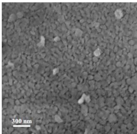
SEM of Alunox™ 70 (primary powder)
