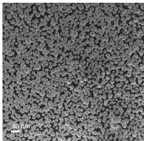
SEM of Alunox™ 70G
